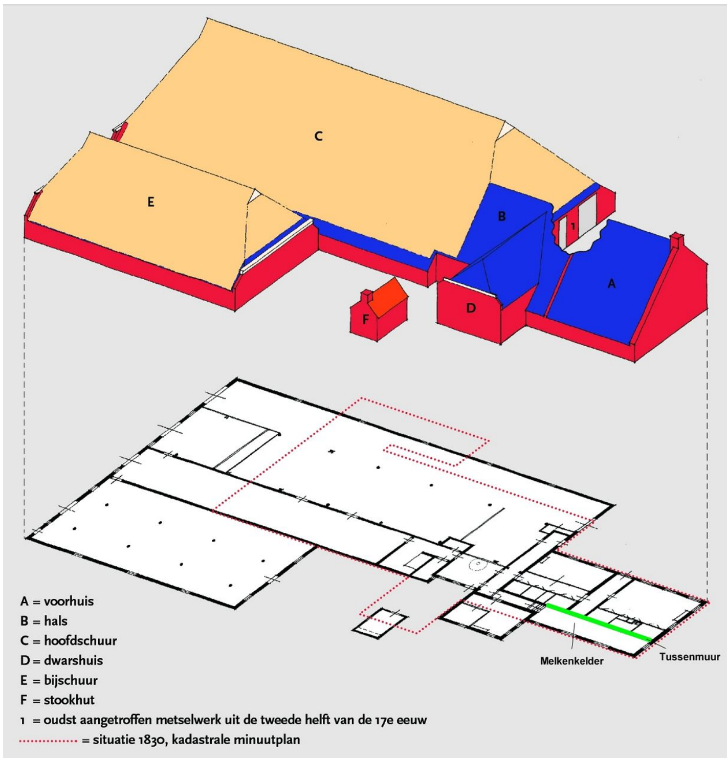
Afbeelding 3.1 Projecttekening van de boerderij Noorddijkerweg 32. De tussenmuur is met een groene lijn aangegeven. Tekening: J.M. Verkerk en Studio van Stralen.
