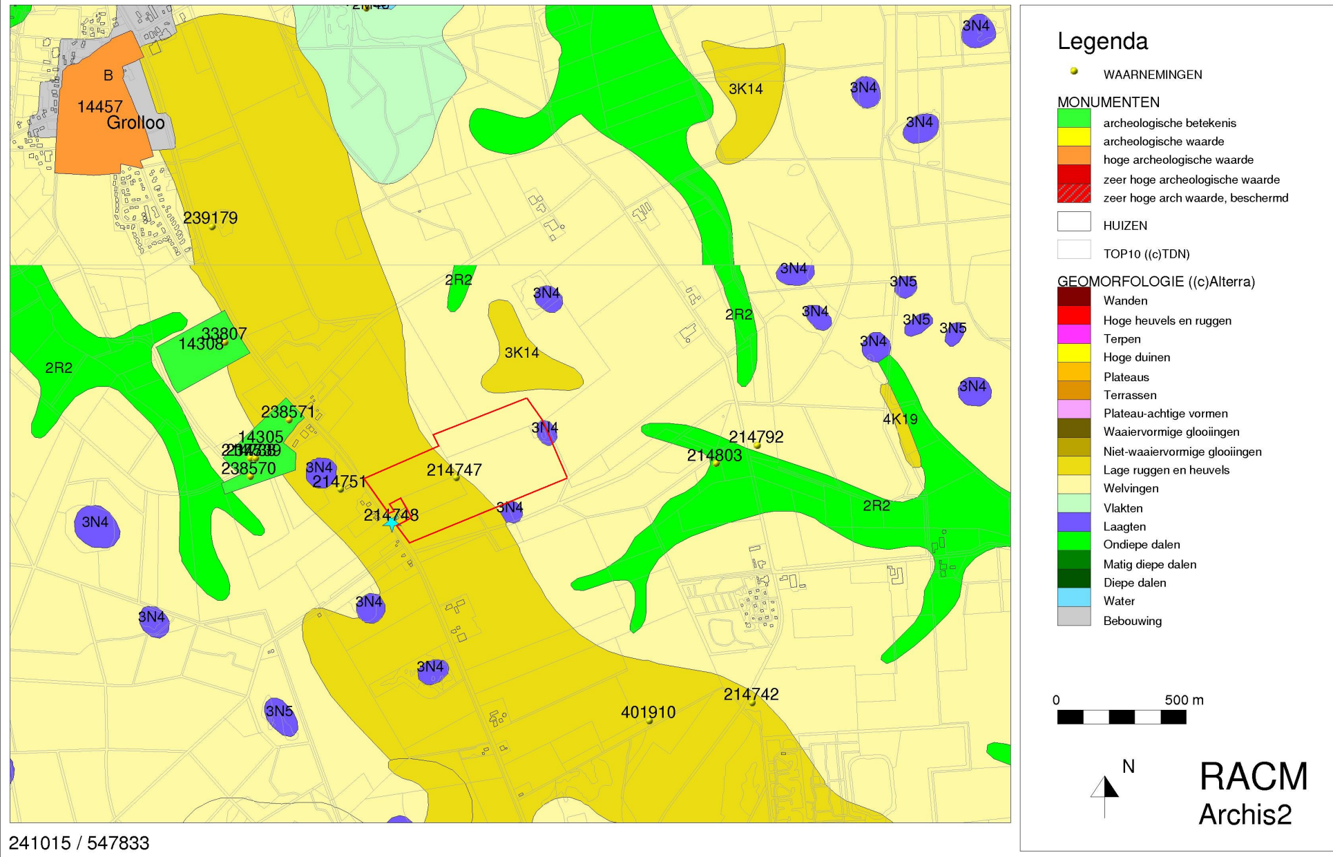
Afbeelding 3 Geomorfologische Kaat van het gebied met monumenten en waarnemingen in de omgeving van de onderzoekslocatie (rood omlind). Bron: Rijksdienst voor Archeologie, Cultuurlandschap en Monumenten (RACM)/Archis II, 22 oktober 2007.
